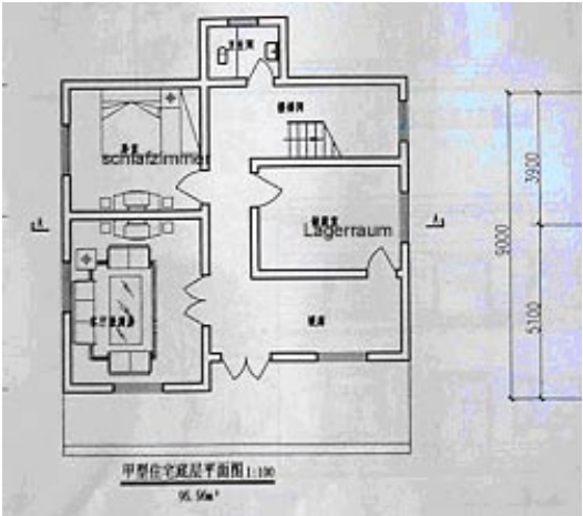
新建建筑平面图
